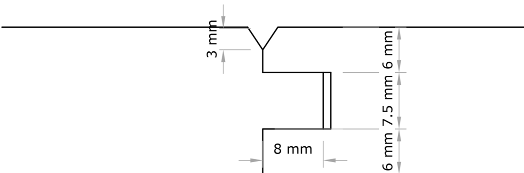
V GROOVE SHADOW
